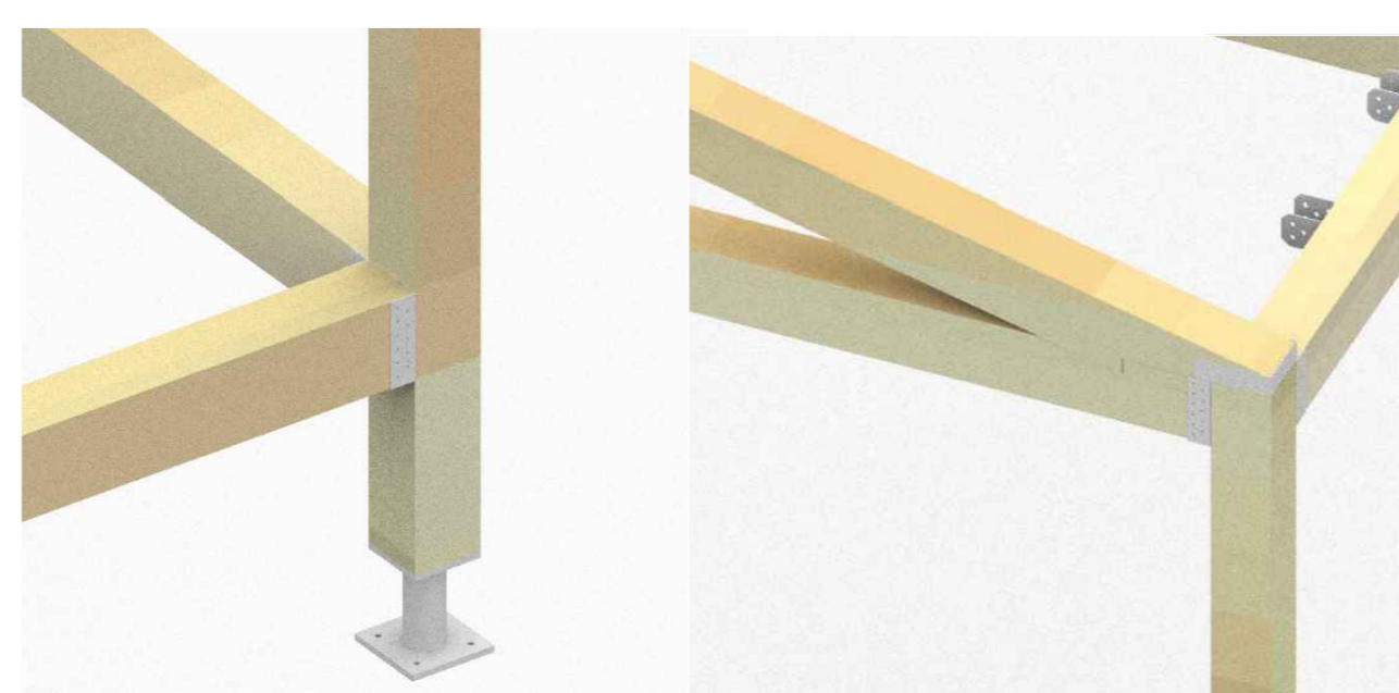
Pillar: Sistema de connexió pilar-forjat
